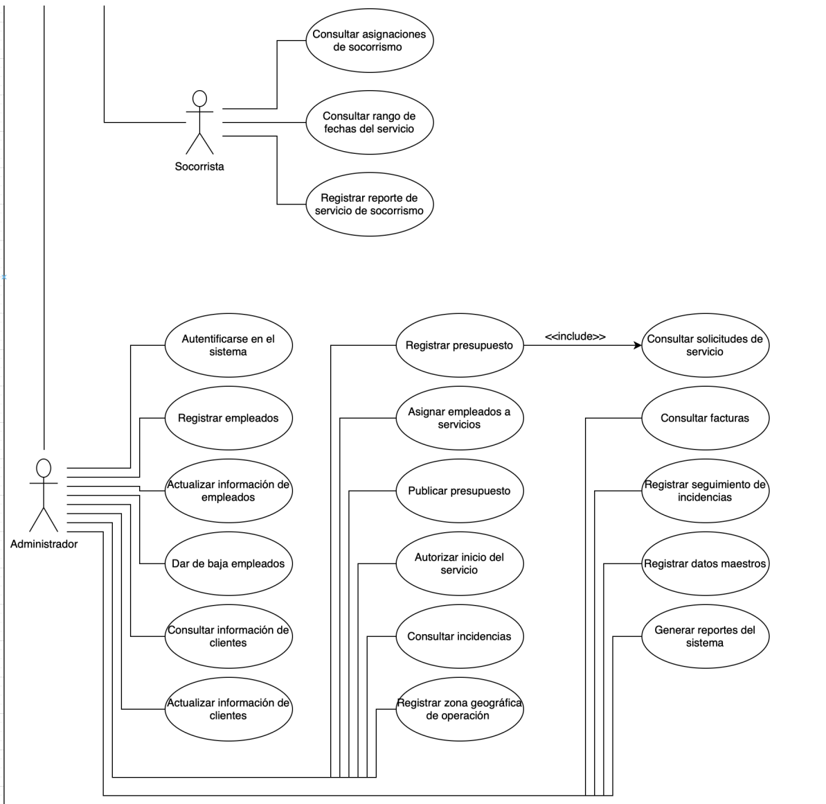
Imagen 1: Diagrama de Casos de Uso
